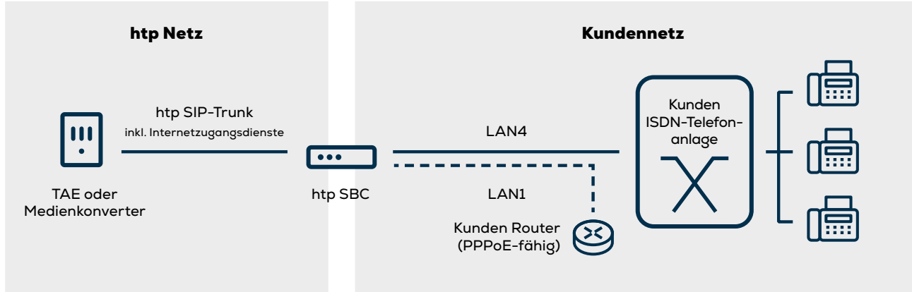
Abb.: SIP-Trunk Kundenanschlusung unter Verwendung eines kundeneigenen Routers
